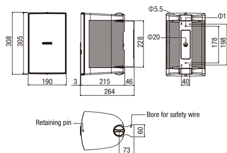
VS6 / VS6W
