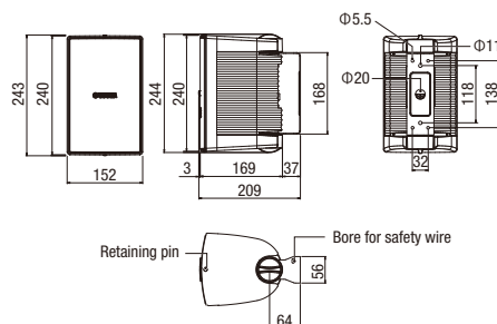
VS4 / VS4W
